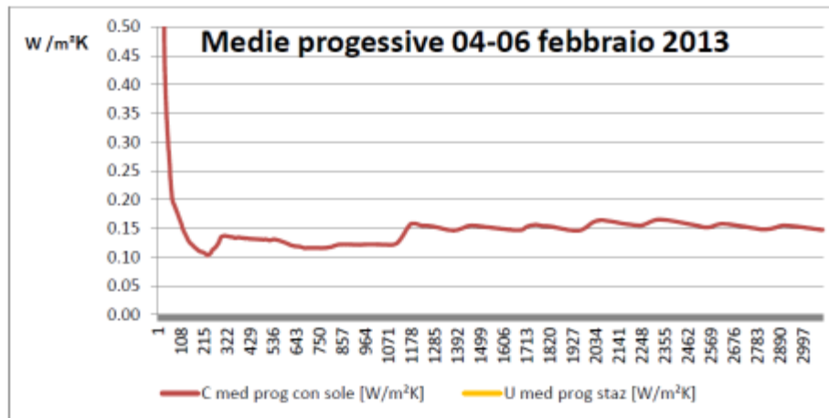
Misure con passo temporale di 10 min per 4 giorni – influenza irraggiamento solare dalla misura 1178.
