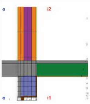
Ponte termico del balcone con muratura in doppio tavolato e cassonetto
