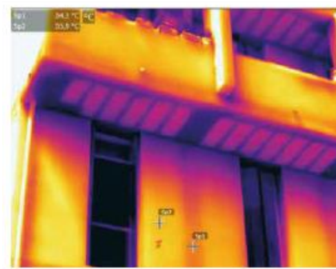
Facciata di edificio, \Delta T = 1,6 \text{ }^\circ\text{C} giugno, esposizione nord-est, pranzo
