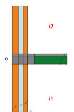
Ponte termico della trave di bordo con muratura in doppio tavolato e intercapedine d'aria
