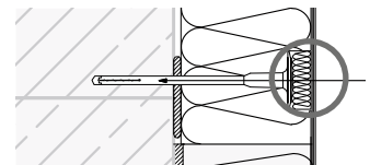
Soluzione ad incasso
