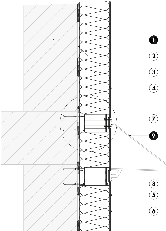
Alternative per i fissaggi
