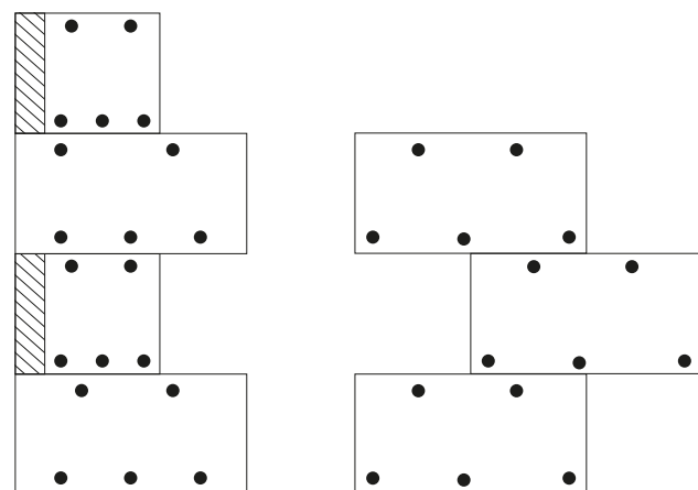
Schema E - Altezza edificio > 10 m
