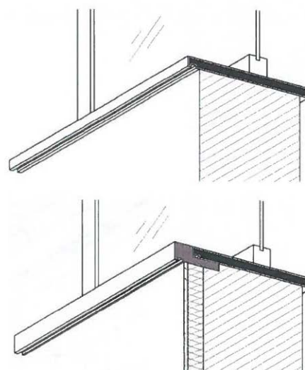
Esempio di prolungamento del davanzale di finestra
