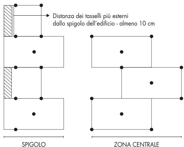
Schema A - Altezza edificio fino a 10 m
