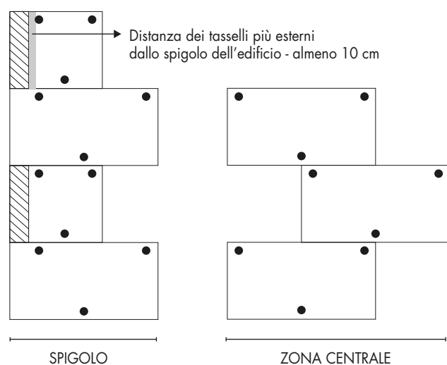
Schema D - Altezza edificio fino < 10 m
